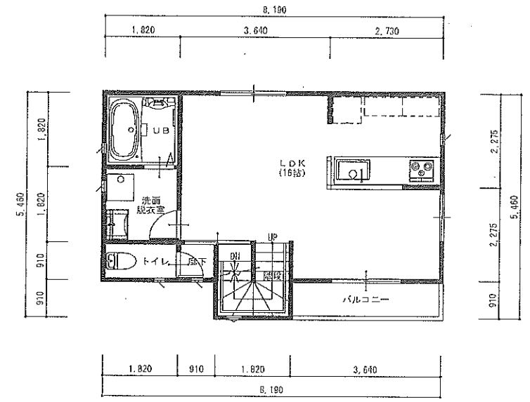
2階 平面図
