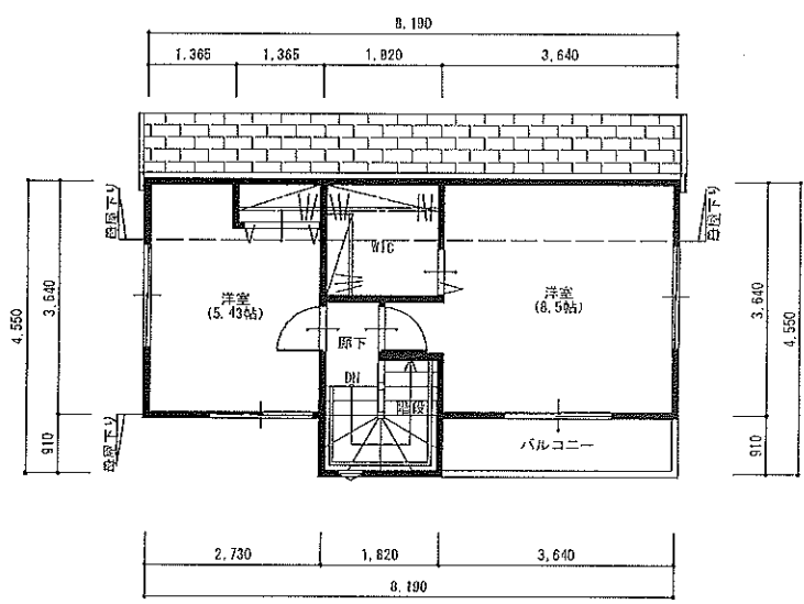
3階 平面図
