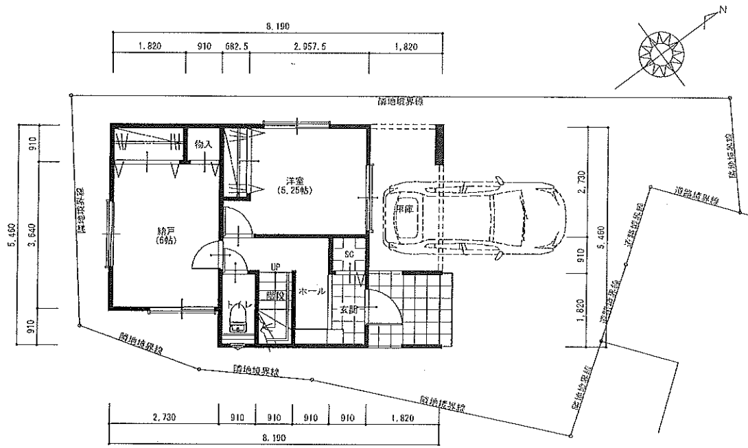
1階 平面図
